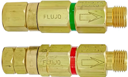
Arrestadoras de flama Código INFRA: 5209
